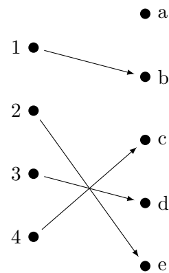
Abbildung 4: Funktion f_3
