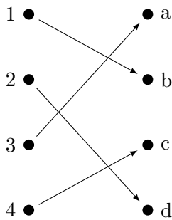
Abbildung 2: Funktion f_1
