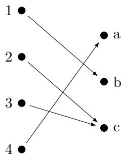
Abbildung 3: Funktion f_2
